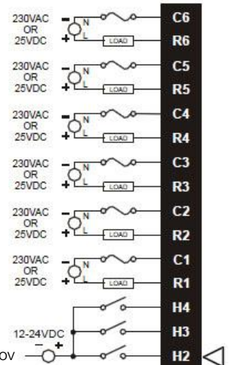
J2 黑色端子 开关量正逻辑输入 / 继电器输出
