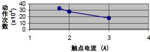
继电器寿命曲线
