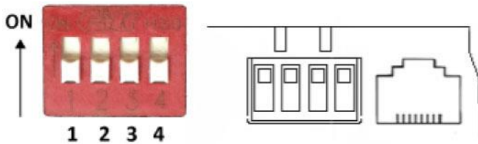
DIP 拨动开关
